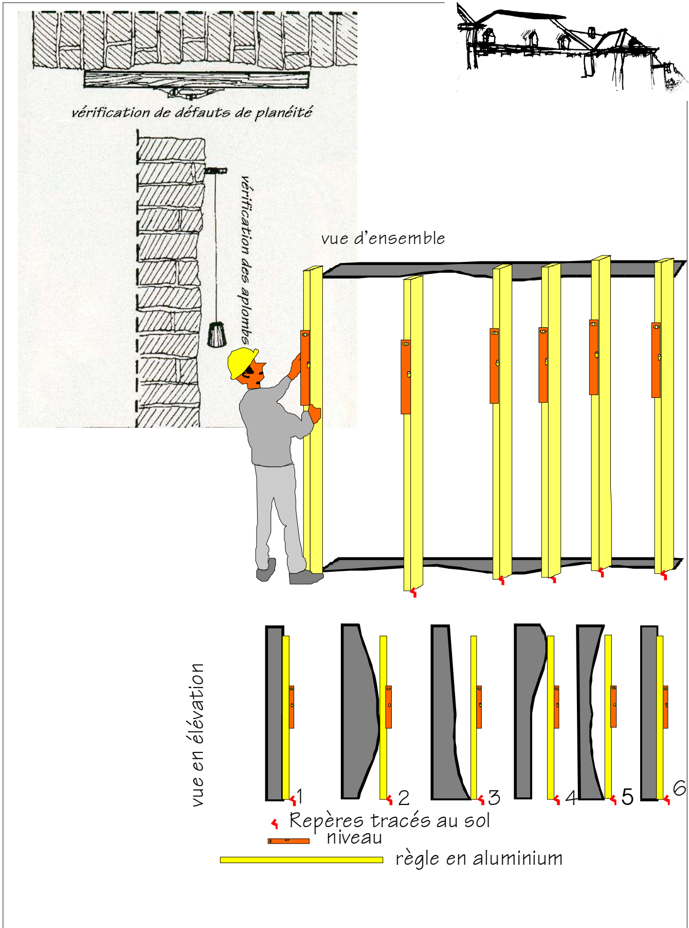
Recherche d'alignement des guides de plafonnage
